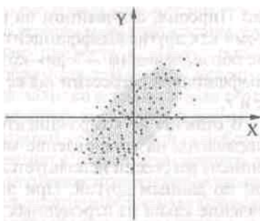
Рис.12.1. Диаграмма рассеивания.
